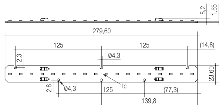
LLE G1 24x280mm 1250lm ADV-SE
