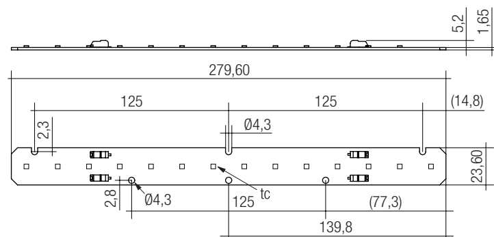
LLE G1 24x280mm 650lm ADV-SE
