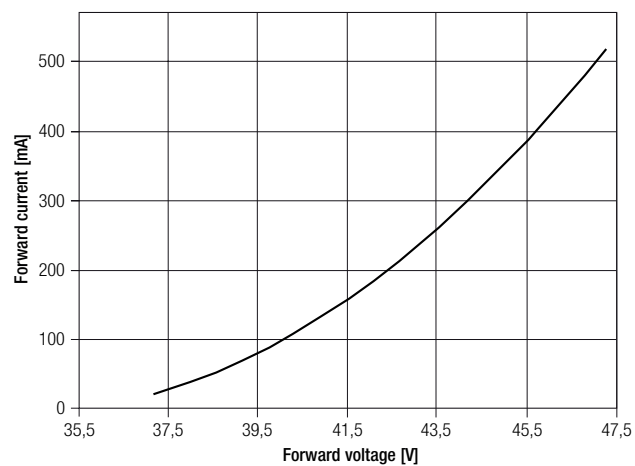
LLE G1 24x560mm 1300lm
