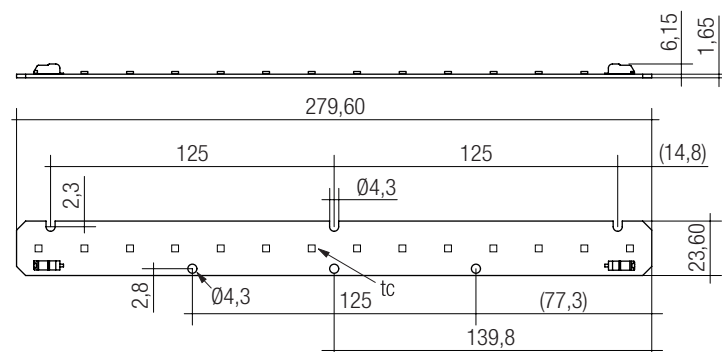
LLE G1 24x280mm 650lm SNC
