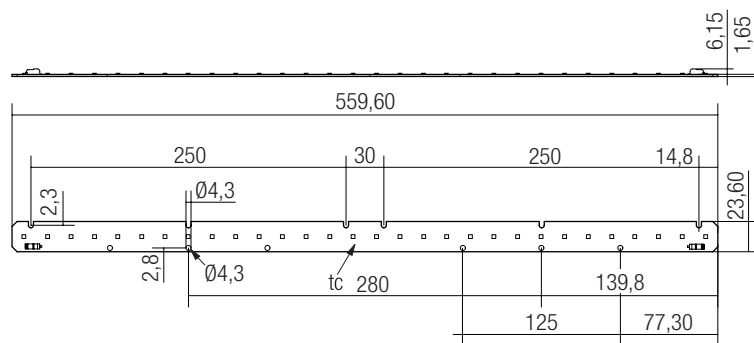
LLE G1 24x560mm 2400lm SNC
