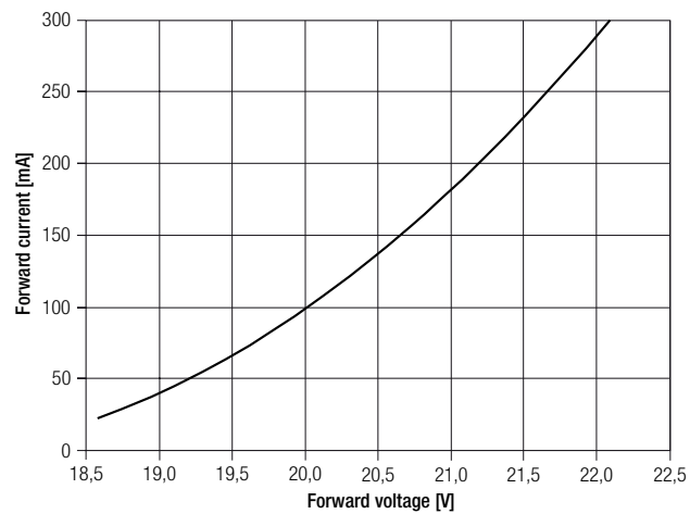
LLE G1 24x280mm 650lm
