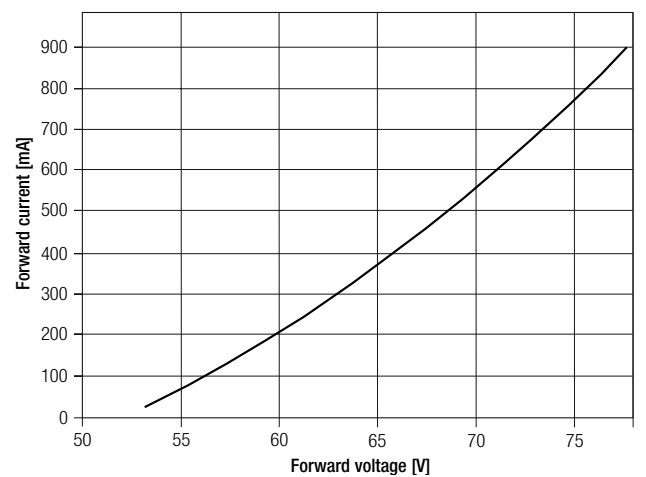
LLE G1 24x560mm 2400lm
