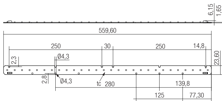
LLE G1 24x560mm 1300lm SNC
