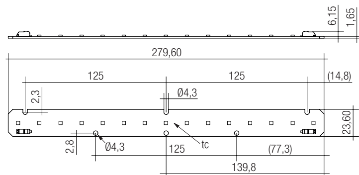
LLE G1 24x280mm 1250lm SNC
